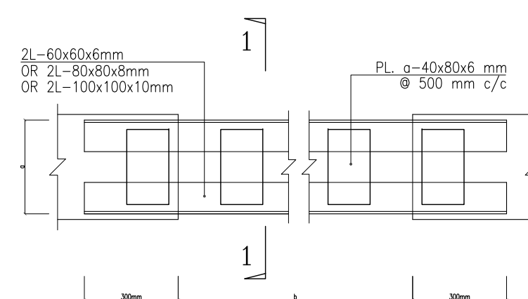
LINTEL PLAN -2L Sc: N.T.S.
