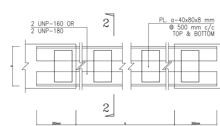
LINTEL PLAN -2 UNP Sci: N.T.S.
