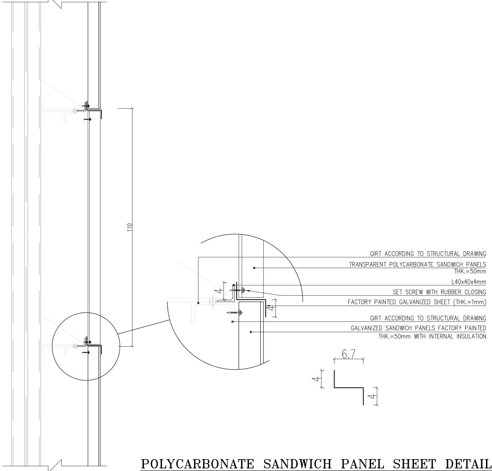
DETAIL-2 Sc:1/10
