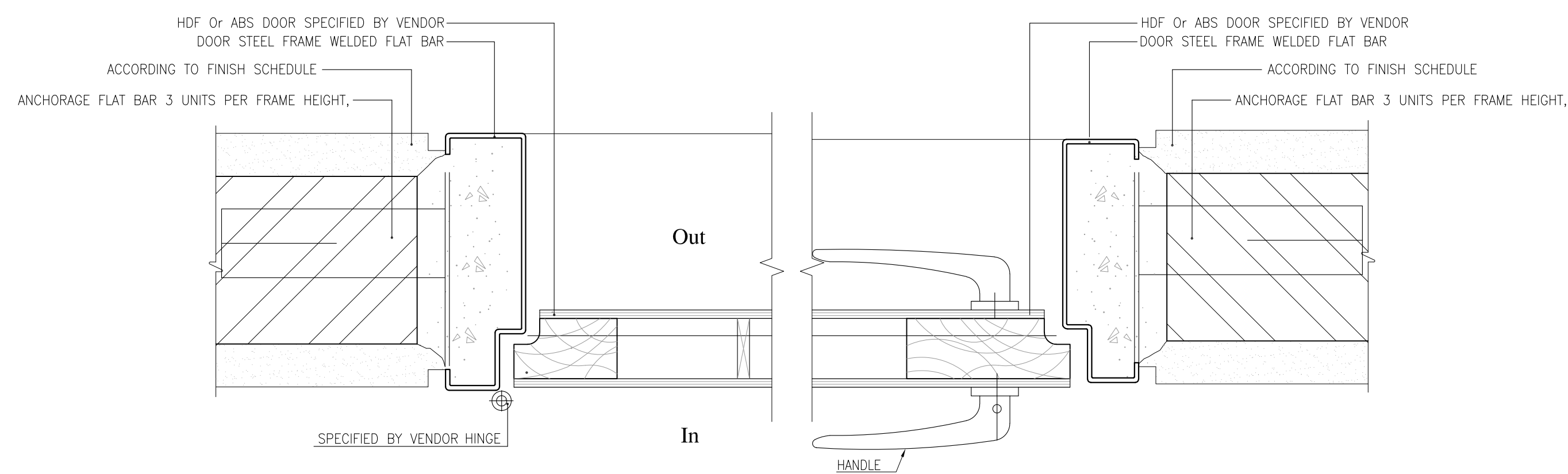
SECTION D-D
